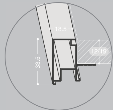
Guide profile
